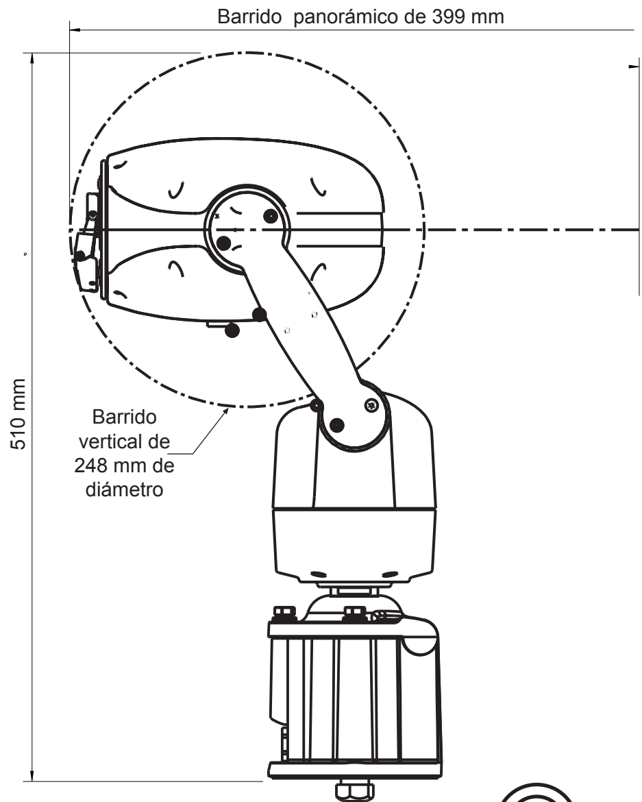
Vista lateral
