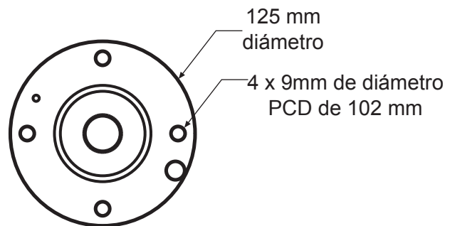
Vista inferior
